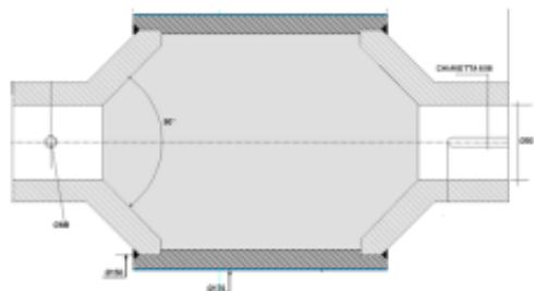
PARTICOLARE "A"
